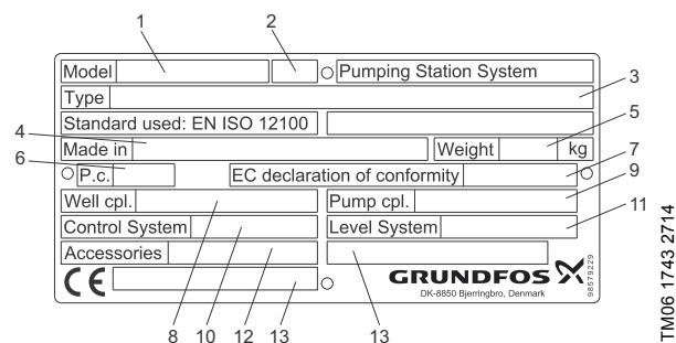
Fig. 2 Typeskilt, PS.S-pumpestationssystemer
