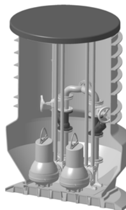
Brønd med to pumper og direkte udløb
