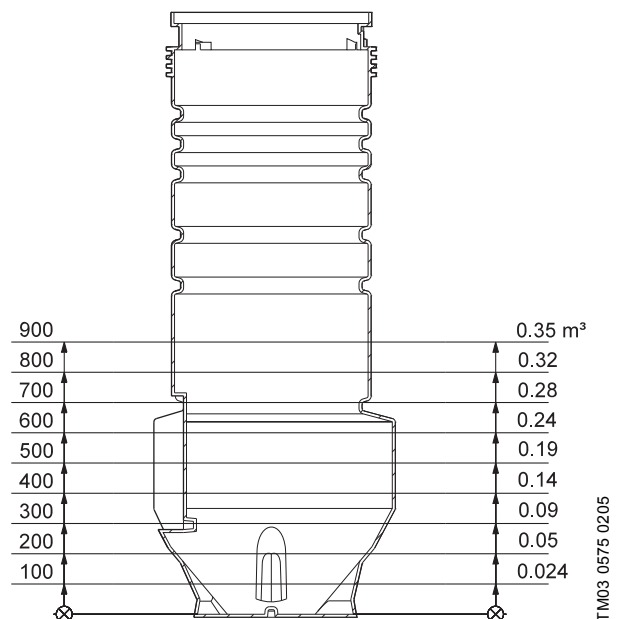
Fig. 25 Effektivt volumen i forhold til niveau, PUST600
