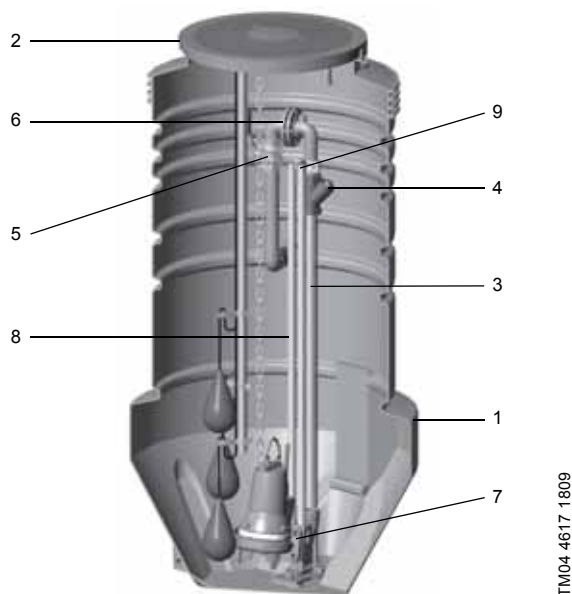
Fig. 9 Små pumpestationer fra Grundfos
