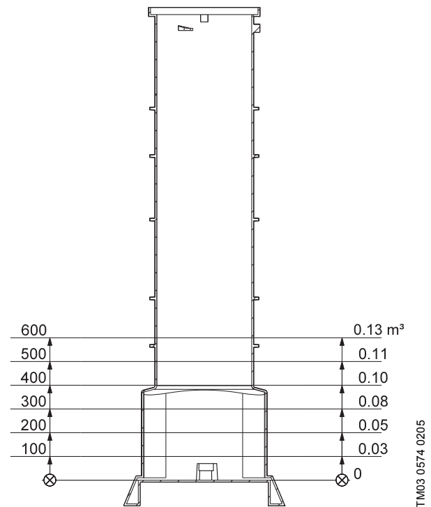
Fig. 24 Effektivt volumen i forhold til niveau, PUST400
