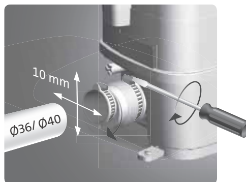
Fig. 17 Højde- og sideopretning mulig ved brug af Ø36/40 tilgangsrør
