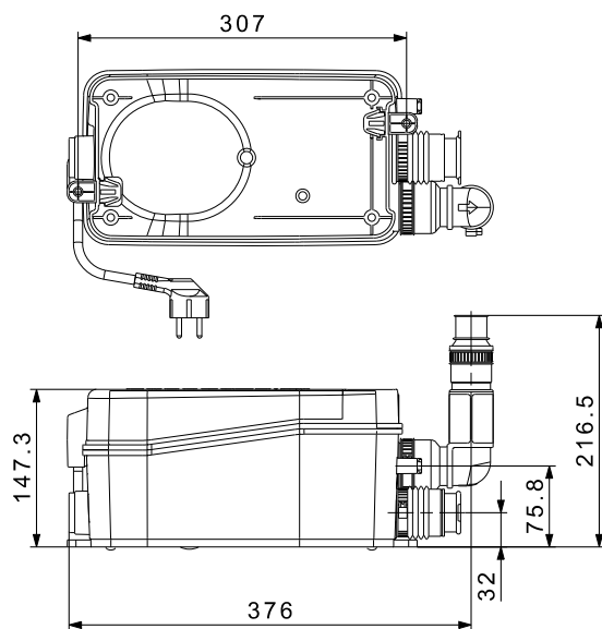
Fig. 44 Måltegninger, Sololift2 D-2
