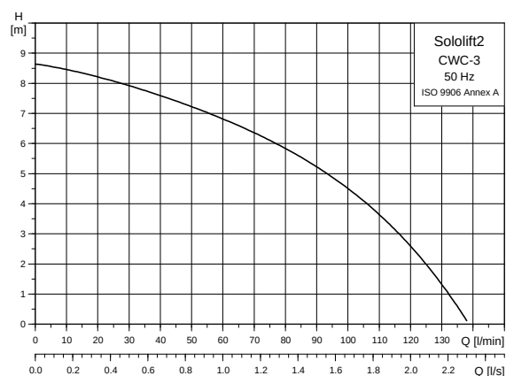
Fig. 26 Ydelseskurver, Sololift2 CWC-3
