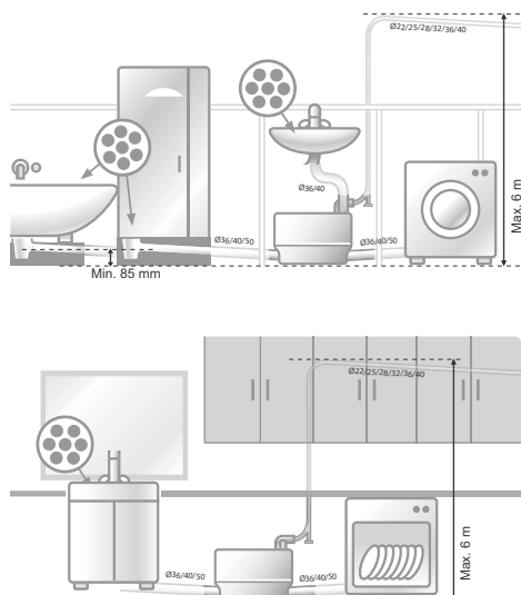
Fig. 31 Installationseksempler
