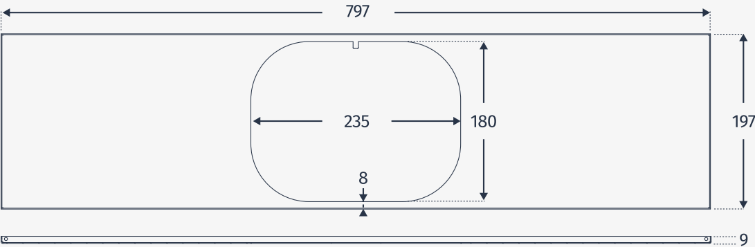
Renne | Frame
